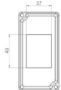
TAMPA P/ 3 INTERRUPTORES HORIZONTAIS 1"
