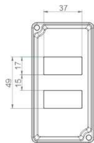
TAMPA P/ 2 INTERRUPTORES HORIZONTAIS SEPARADOS 1"
