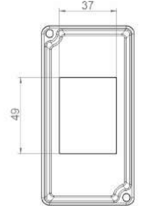
TAMPA P/ 3 INTERRUPTORES HORIZONTAIS 1"
