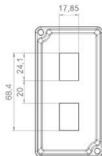
TAMPA P/ 2 RJ S/MOLDURA 1"
