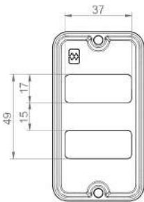
TAMPA P/ 2 INTERRUPTORES HORIZONTAIS SEPARADOS 1/2" E 3/4"
