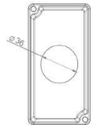
TAMPA P/ 1 TOMADA REDONDA 1"
